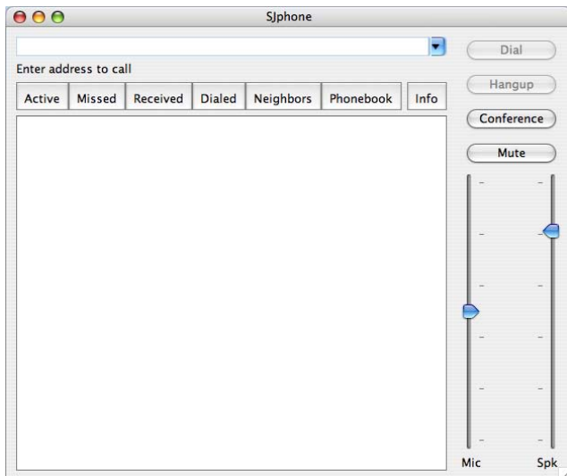
Fig.1 - Fenêtre principale
