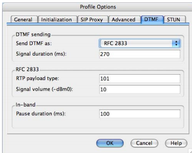
Fig.7 - Réglages DTMF
